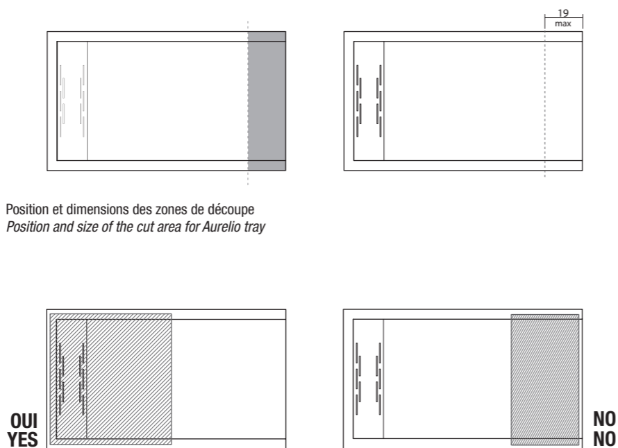
Zone conseillée pour la position de la pomme de douche Suggestions for installation of shower head
