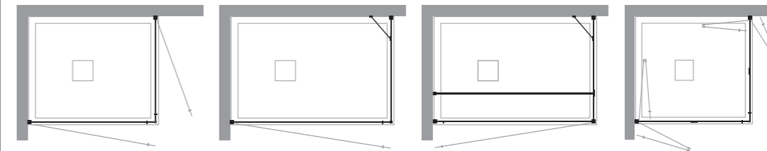
MI-PBA + MI-PBA MI-PBA + MI-F MI-PBA + MI-FA [*] MI-PSO + MI-PSO
