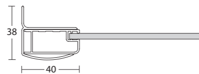
Art. 160 profilé mural + Art. 207 montant vertical Art. 160 wall profile + Art. 207 vertical profile pour/for CO : PGI - PGI2 - PSC3 - PSC - PSO - PSC2 - VSC
