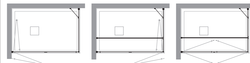
MI-PSO + MI-F MI-PSO + MI-FA [*] MI-PSA2 + MI-FA [*]
