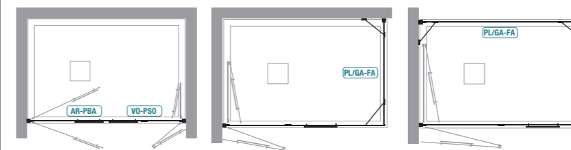
VO-PSO + AR-PBA [*] VO-PSO + VO-F + PL-FA (*) VO-PSO + VO-F + PL-FA (*)
