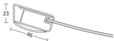
Art. 090 profilé mural + Art. 207 montant vertical Art. 090 wall profile + Art. 207 vertical profile pour/for CO : T61
