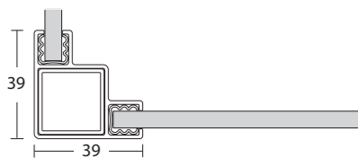
Art 1207 profilé d'angle deux voies + art 1208 télescopique Art 1207 two ways corner connection + art 1208 telescopic
