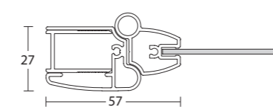
Art. 106 profilé mural + Art. 197 montant vertical + Art. 195 profilé vertical / charnière Art. 106 wall profile + Art. 197 vertical profile + Art. 195 vertical pivoting profile pour/for CO : SVF
