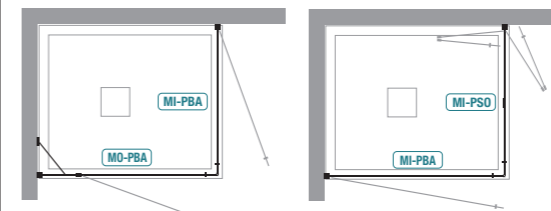
MI-PBA + MO-PBA (*) MI-PBA + MI-PSO
