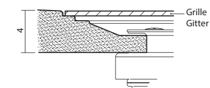
Section du receveur Aurelio avec bonde Section of Aurelio shower tray with waste
