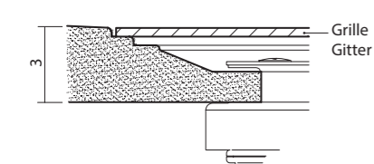
Section du receveur Arturo sans bords avec bonde Arturo shower tray section, waste included
